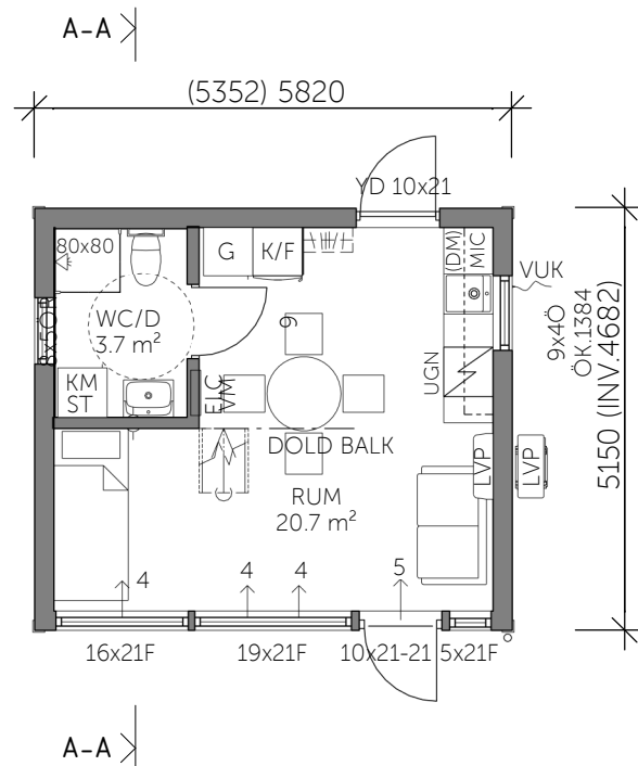
ENTRÉPLAN BOAREA (BOA) 25.1 m 2 BYGGYTA (BYA) 30.0 m 2
